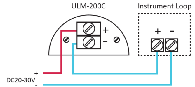
〈系统接线图〉
