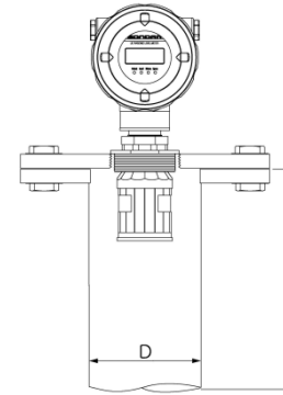
不同内径的加接管及适宜管长 (单位:mm)
